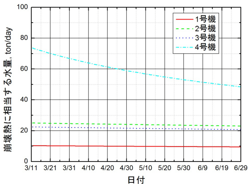
図 11 使用済み燃料棒貯蔵プール内の燃料棒の発熱量に相当する水量
