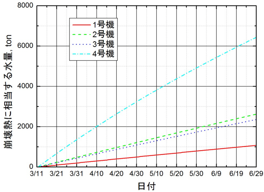
図 13 使用済み燃料棒貯蔵プール内燃料棒の総発熱量に相当する水量
