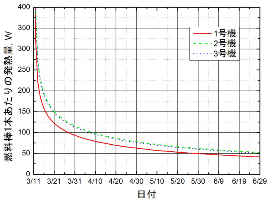
図 5 燃料棒一本あたりの発熱量の経時変化
