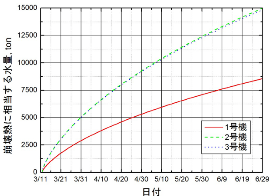
図 9 原子炉停止からの総崩壊熱量に相当する水量
