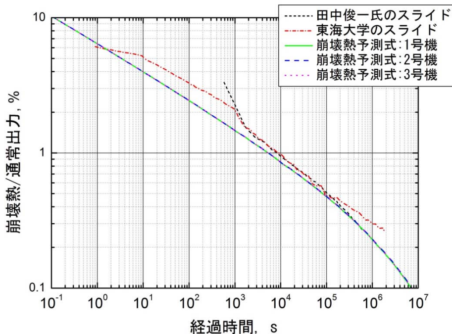
図 3 崩壊熱予測式と他の公表データとの比較[8][9]
