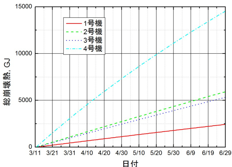
図 12 使用済み燃料棒貯蔵プール内燃料棒の総発熱量
