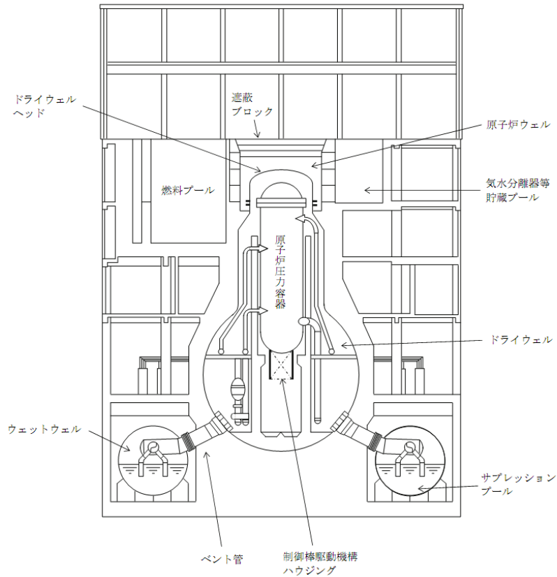
図 1 BWR3 マーク I 型原子炉建屋概要図[3]
