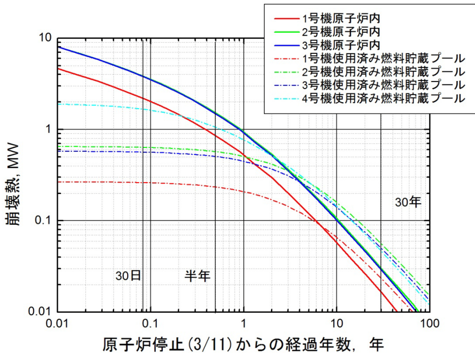
図 14 長期間にわたる崩壊熱の経時変化
