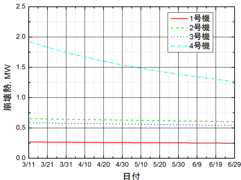
図 10 使用済み燃料棒貯蔵プール内の燃料棒の発熱量の変化
