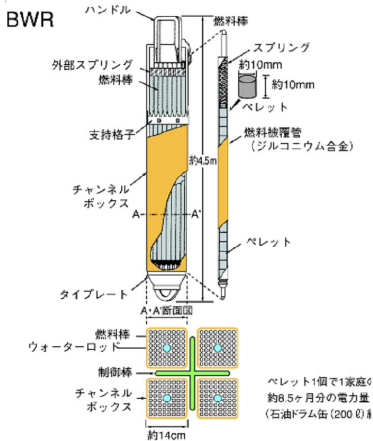
図 2 燃料集合体および燃料棒の概略図[4]
