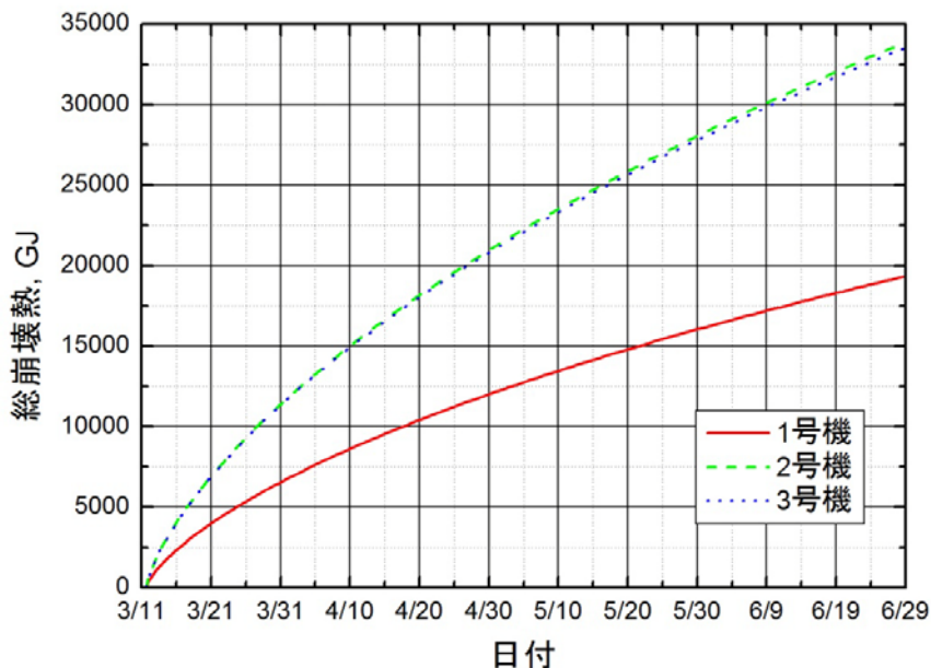
図 8 原子炉停止からの総崩壊熱量
