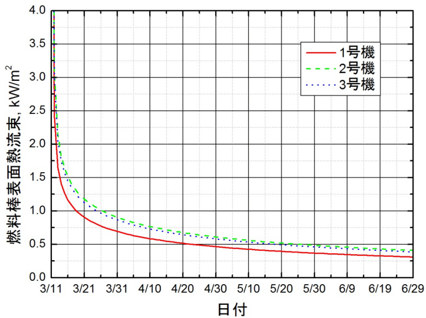
図 6 燃料棒表面の熱流束の経時変化
